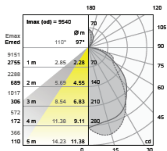
FOTOMETRÍA 6 X 54 W
