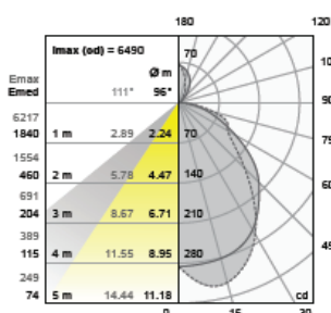
FOTOMETRÍA 4 X 54 W
